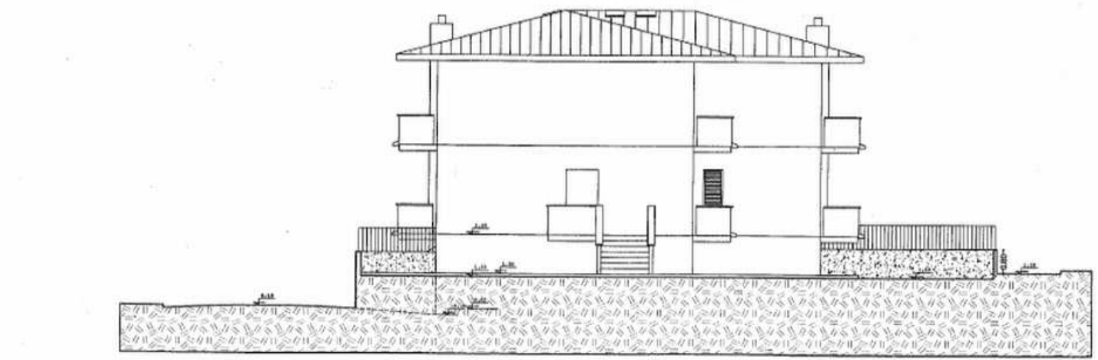
PROSPETTO ③ LATO NORD
