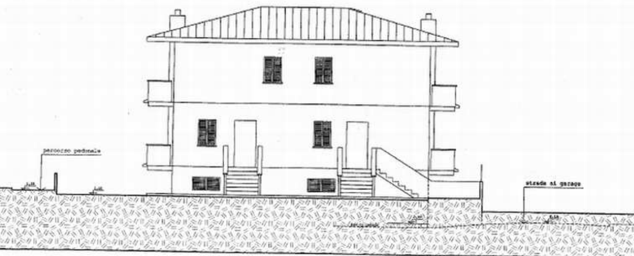
PROSPETTO SUD
