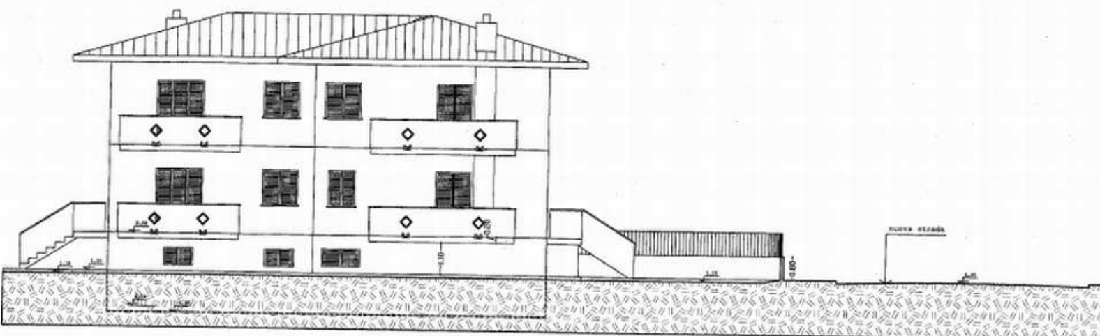
PROSPETTO OVEST
