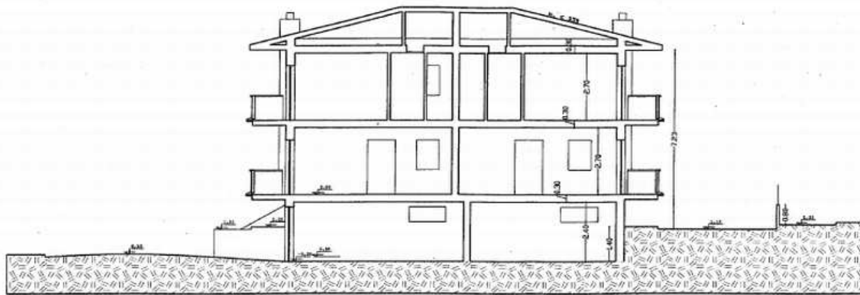
sez. A-A'
